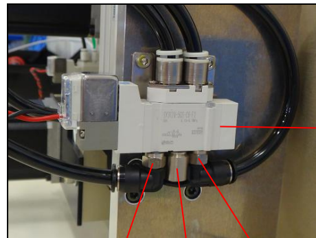
カッター用エアソレノイド
