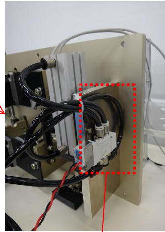
カッター用エアソレノイド
