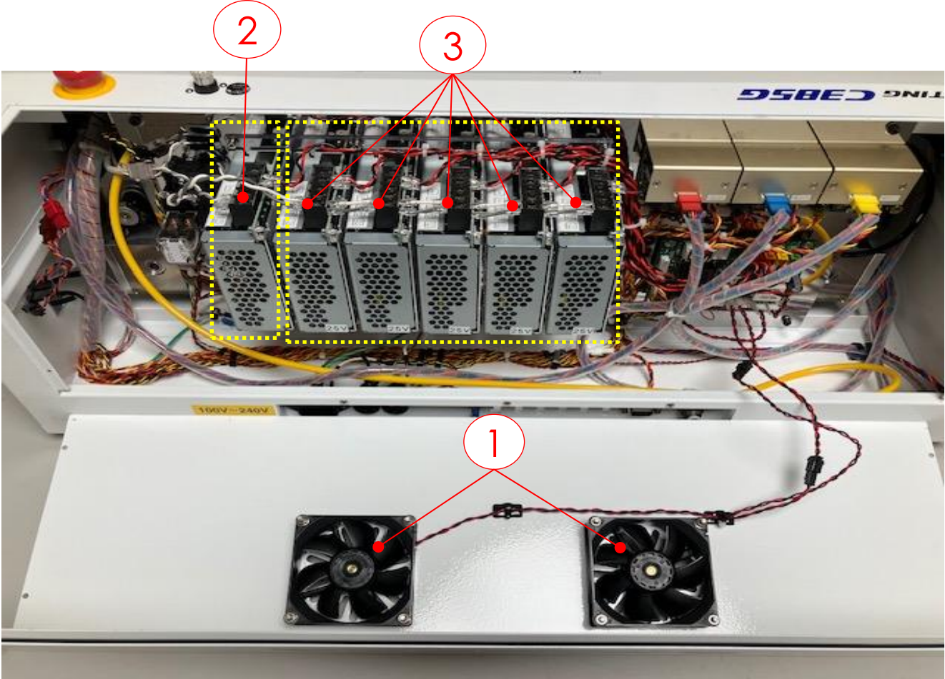
C385G 内部 (1)
