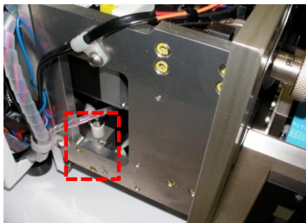
ロールアップ用ソレノイド (左/右) ソレノイドの加工以外同じ
