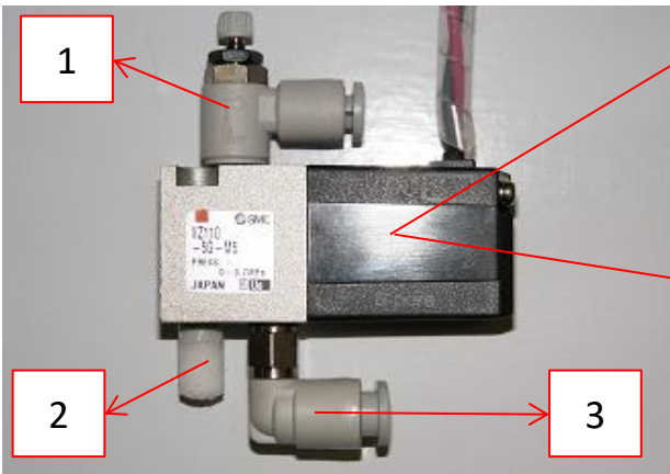
ロールアップ用ソレノイド (左/右) ソレノイドの加工以外同じ
