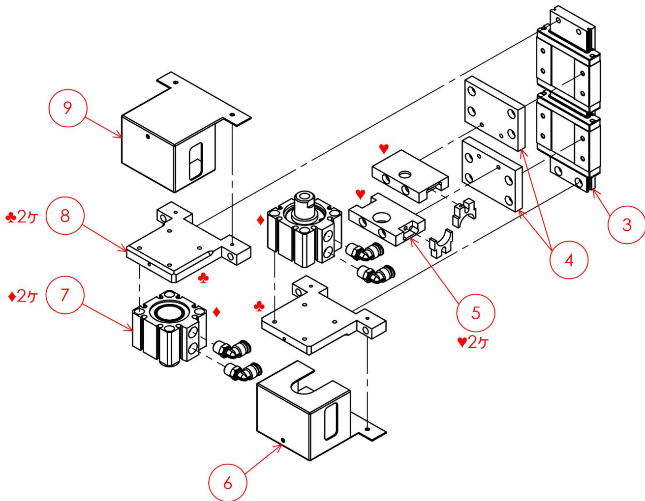
エアカッターブロック(2)
